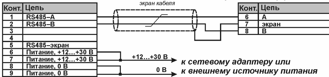
Рисунок 3 – Схема подключения ПДУ к преобразователям частоты
