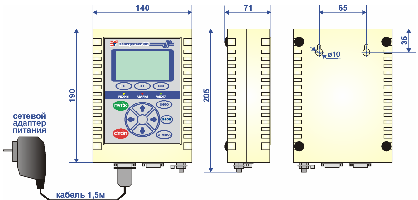
Рисунок 1 – Габаритные и установочные размеры ПДУ
